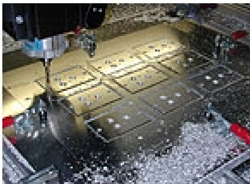
Fräsen von Aluminium - Frontplatten
